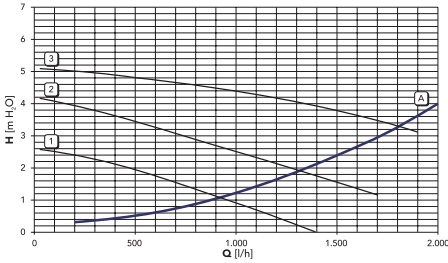
Şek.16 - Sirkülör yük / basınç kayıpları
