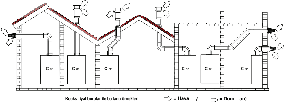
Koaksiyal borular ile bağlantı
