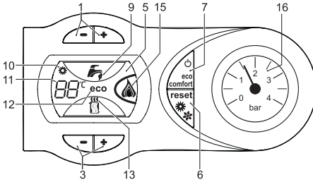
Şek.1 Kontrol paneli
