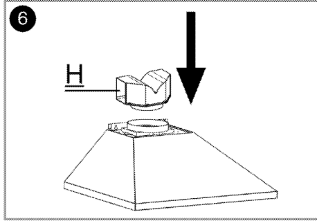
Şekil 6'da gösterildiği gibi hava yönlendiricisi H yerine takılır.
